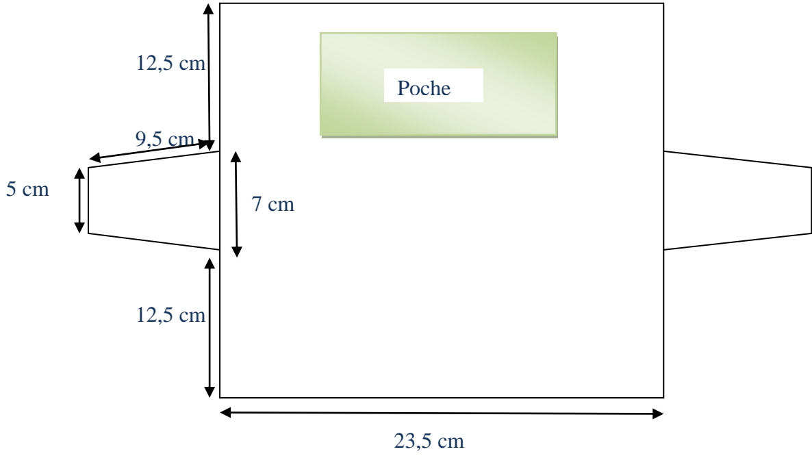
Schéma avec coutures comprises de 0,7 cm
